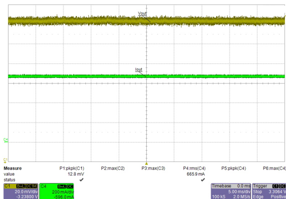
Fig 8. I_{OUT} = 700\text{mA}
