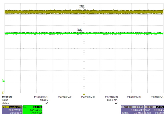
Fig 10. I_{OUT} = 900\text{mA}
